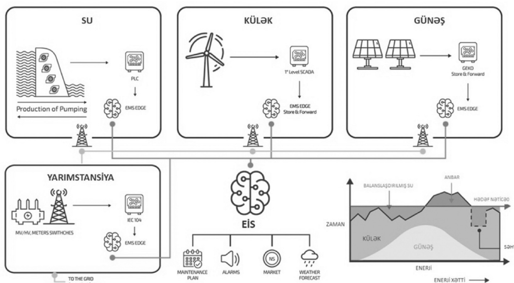
Şəkil 3. Enerji İdarəetmə Sistemi
