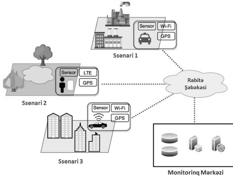
Şəkil 6. Ətraf Mühitin Monitoring Sistemləri təsviri
