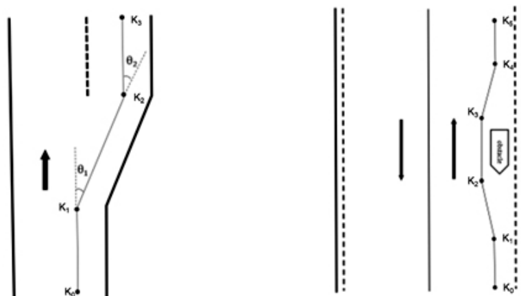
Şəkil 7. Sərhəd naryadı trayektoriyasında kiçik əyrilərin diaqramı: (a) zolaqların dəyişdirilməsi; (b) maneələrdən qaçmaq.
