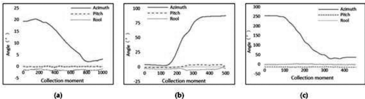
Şəkil 3. Təhlükəli keçid prosesi zamanı istiqamət sensorunun üçoxlu məlumatlarının dəyişməsi: (a) 20° sola təhlükəli keçid; (b) sağa 90° təhlükəli keçid; (c) 180° təhlükəli keçid.
